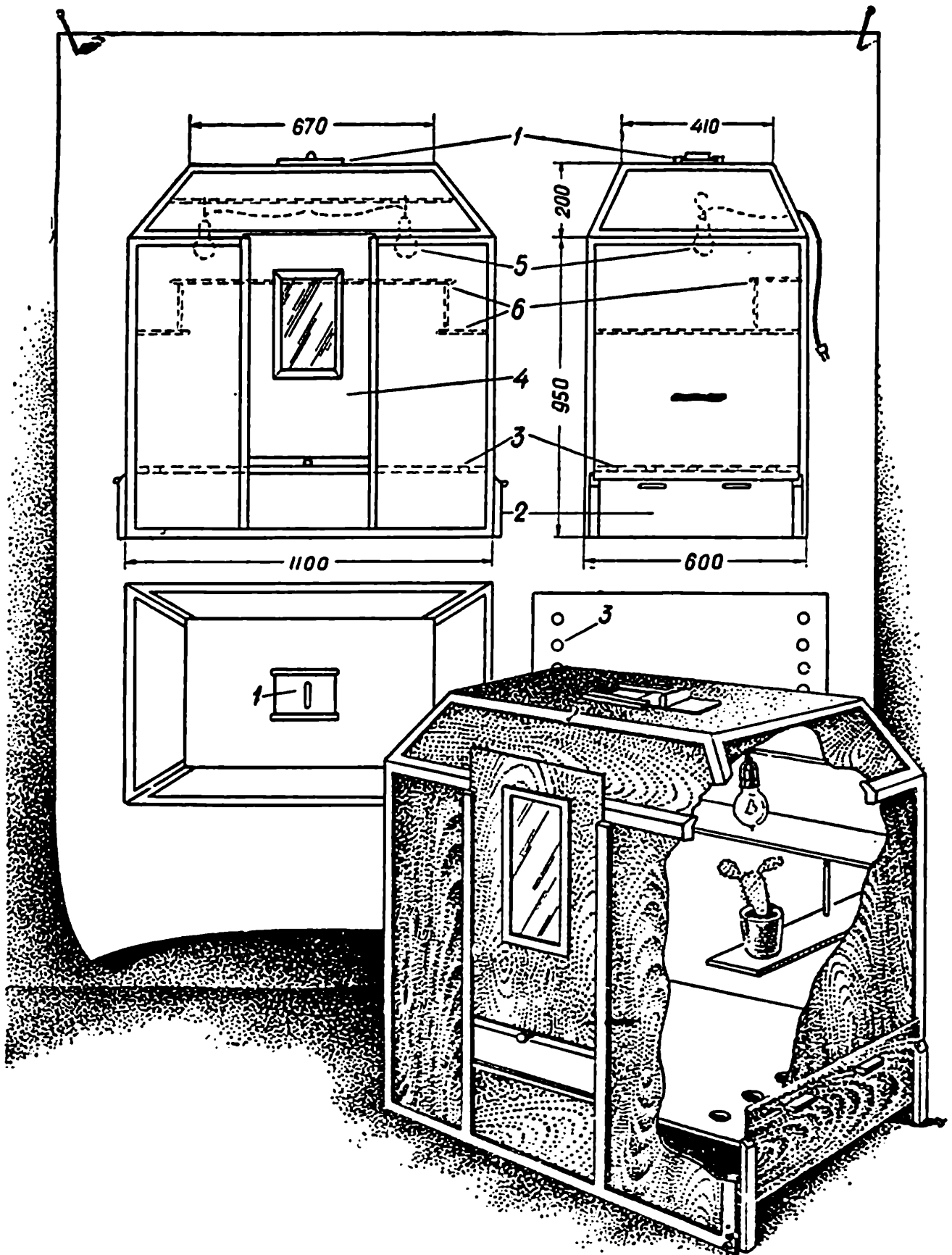
Электрокамера Н. М. Верзилина и ее чертёж с указанием размеров в миллиметрах:
